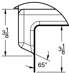
Return Flange
