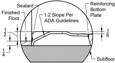
No-Recess
