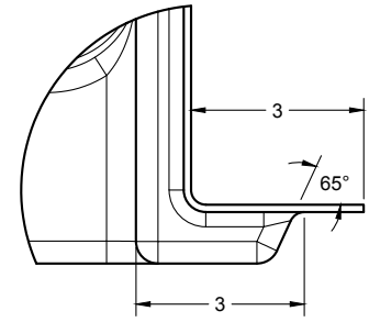
Return Flange
