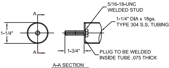
(QNS) NO FLANGE, FIXED STUD DETAIL
