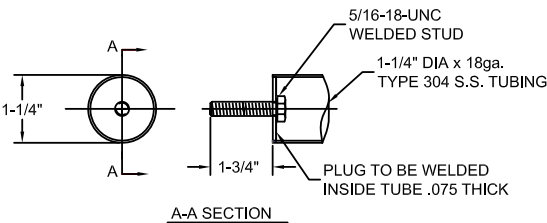
(QNS) NO FLANGE, FIXED STUD DETAIL
